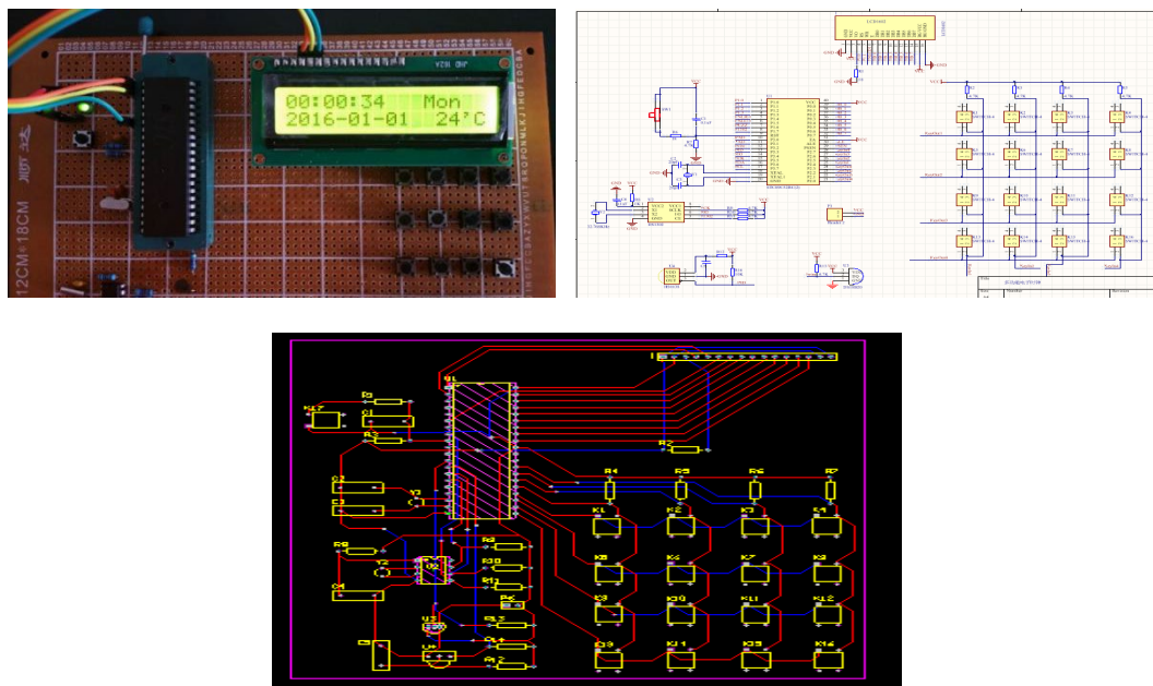
图 15 单片机应用综合实习
